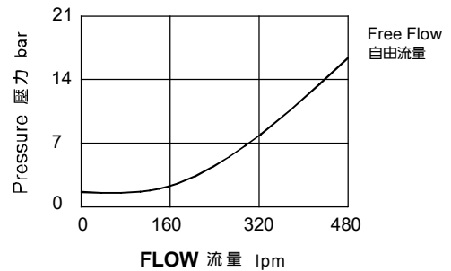
特性曲線
